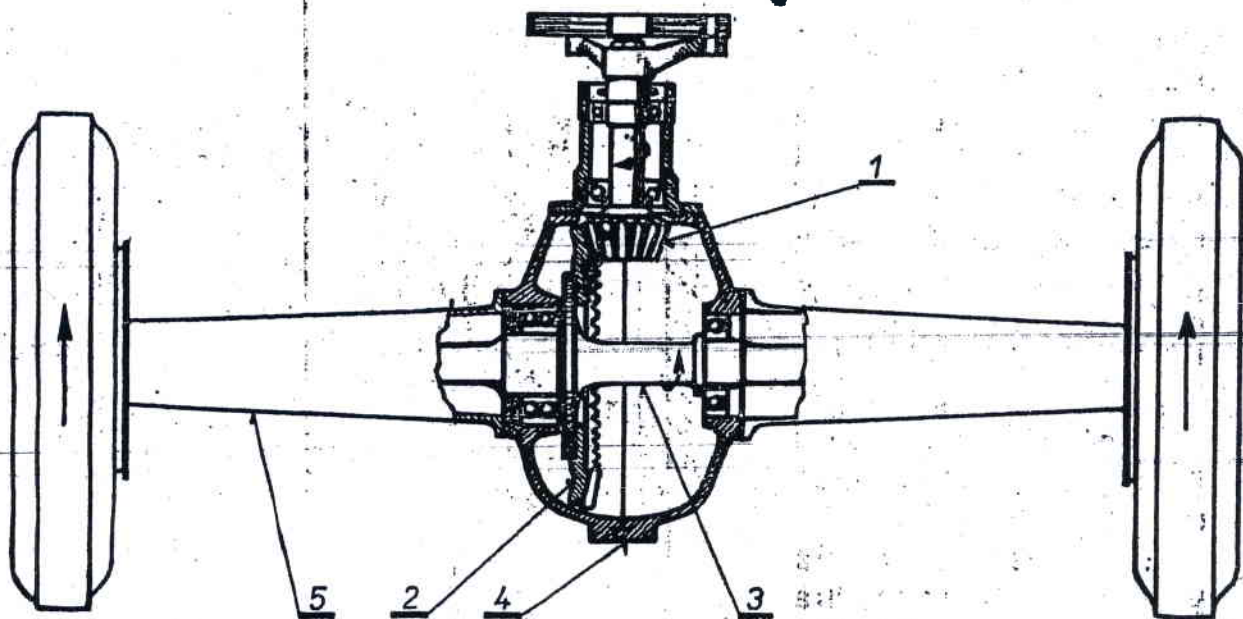
Obr. 47. Zadní náprava s kuželovým stálým převodem s rovnými zuby (bez diferenciálu): 1 — pastorek, 2 — talířové kolo (tzv. redukční soukolí), 3 — hřídel zadních kol, 4 — skříň zadní nápravy, 5 — dutý nosník (trouba)
