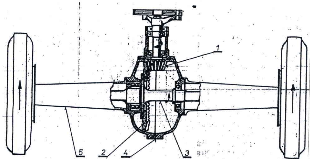
Obr. 47. Zadní náprava s kuželovým stálým převodem s rovnými zuby (bez diferenciálu): 1 — pastorek, 2 — talířové kolo (tzv. redukční soukolí), 3 — hřídel zadních kol, 4 — skříň zadní nápravy, 5 — dutý nosník (trouba)
