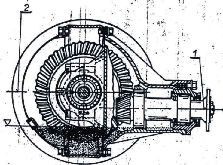
Obr. 48. Hypoidní kuželové soukolí hnací nápravy: 1 — osa pastorku, 2 — osa talířového kola
